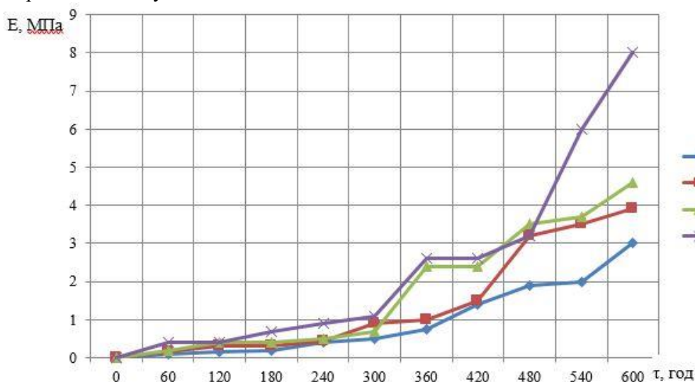
Рис. 2. Міцність газобетонного масиву в залежності від виду сировинної суміші: 1 – цементно-піщаний газобетон; 2 – цементно-золинний газобетон; 3 – цементно-золинний газобетон з доданням Na 2 SO 4 (1%); 4 – цементно-золинний газобетон з доданням NaCl (1%)
